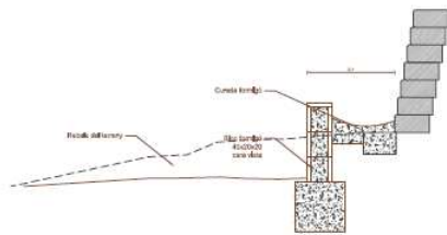
PLANTA I SECCIÓ DEL MUR/BANC I RECOLLIDA D'AIGÜES D'ESCORRENTIA
